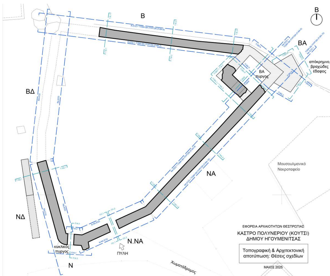
Εικ. 18 Κάτοψη κάστρου Πολυνερίου: θέσεις ζητούμενων σχεδίων όψεων και τομών.
